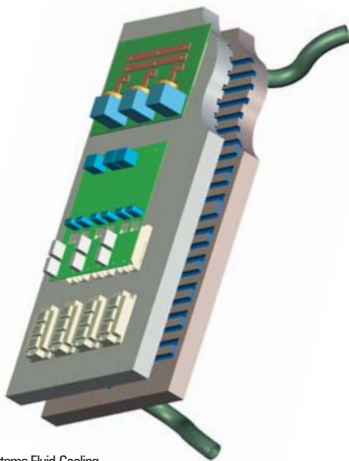
► Sistema Fluid-Cooling.
